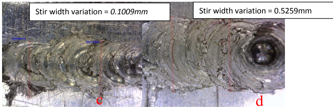
Fig3: Friction stir width variation at (a) 1000rpm (b) 1100rpm (c) 1200rpm (d) 1400rpm
